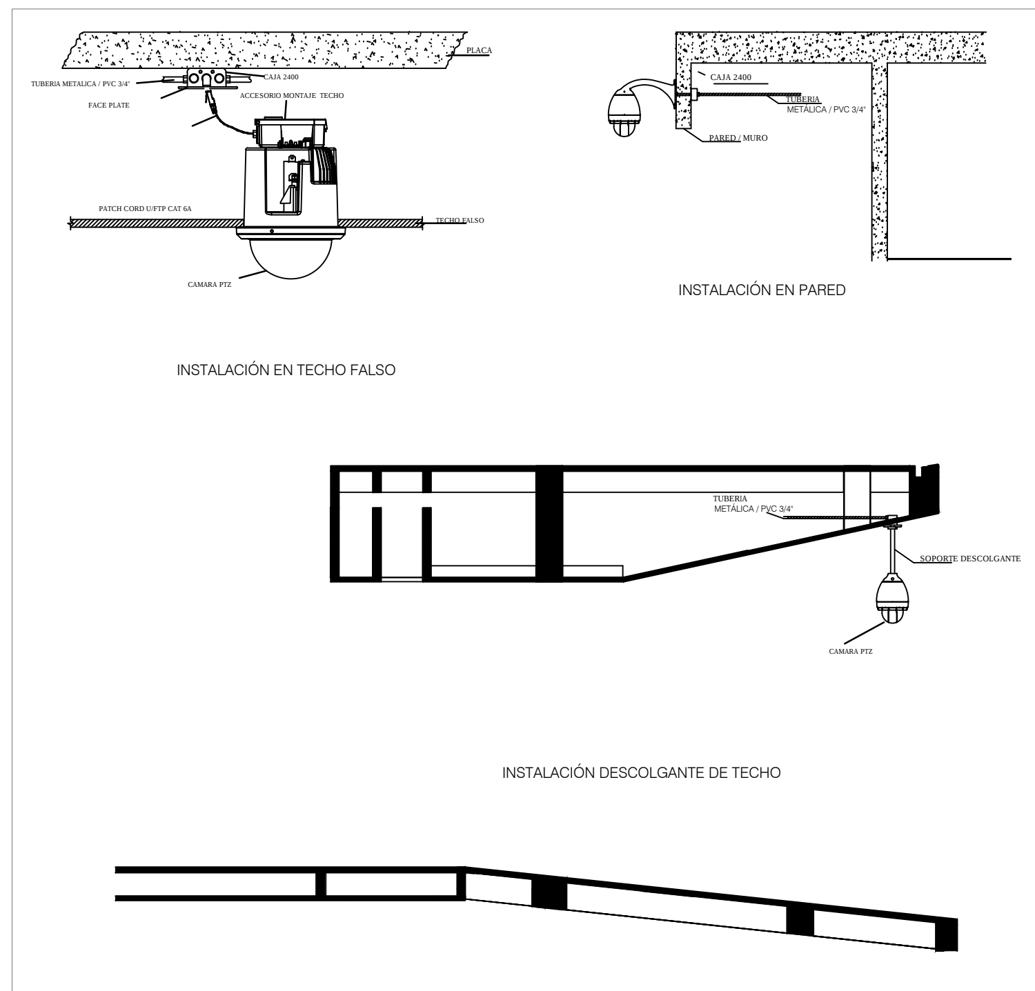
CAMARA TIPO PTZ
