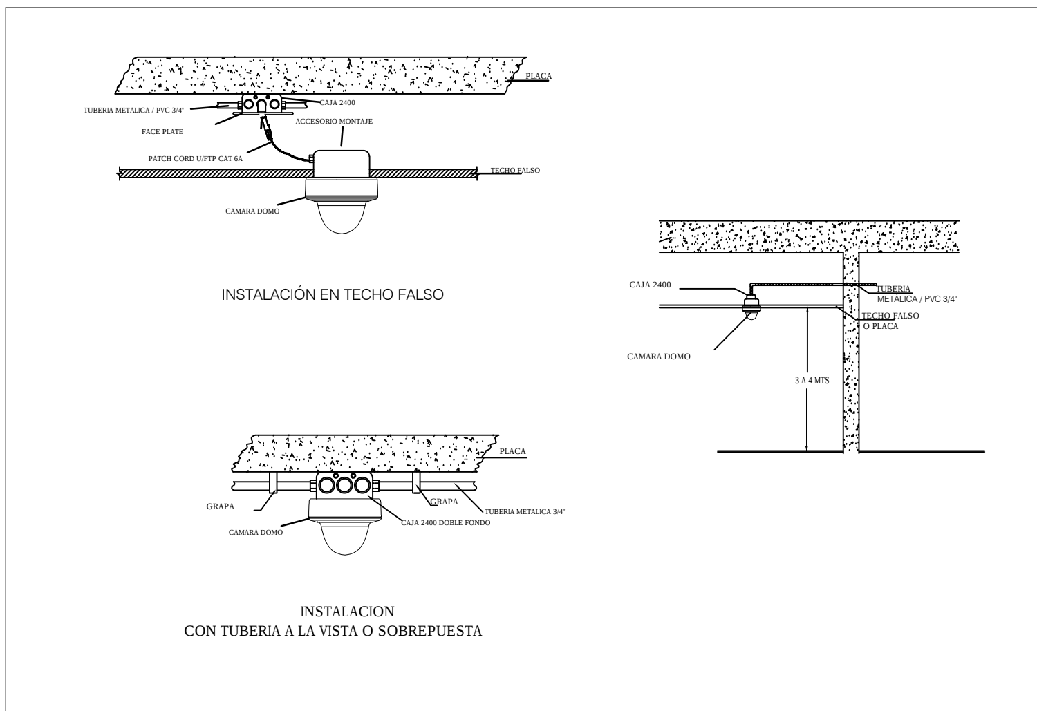
CAMARA TIPO DOMO
