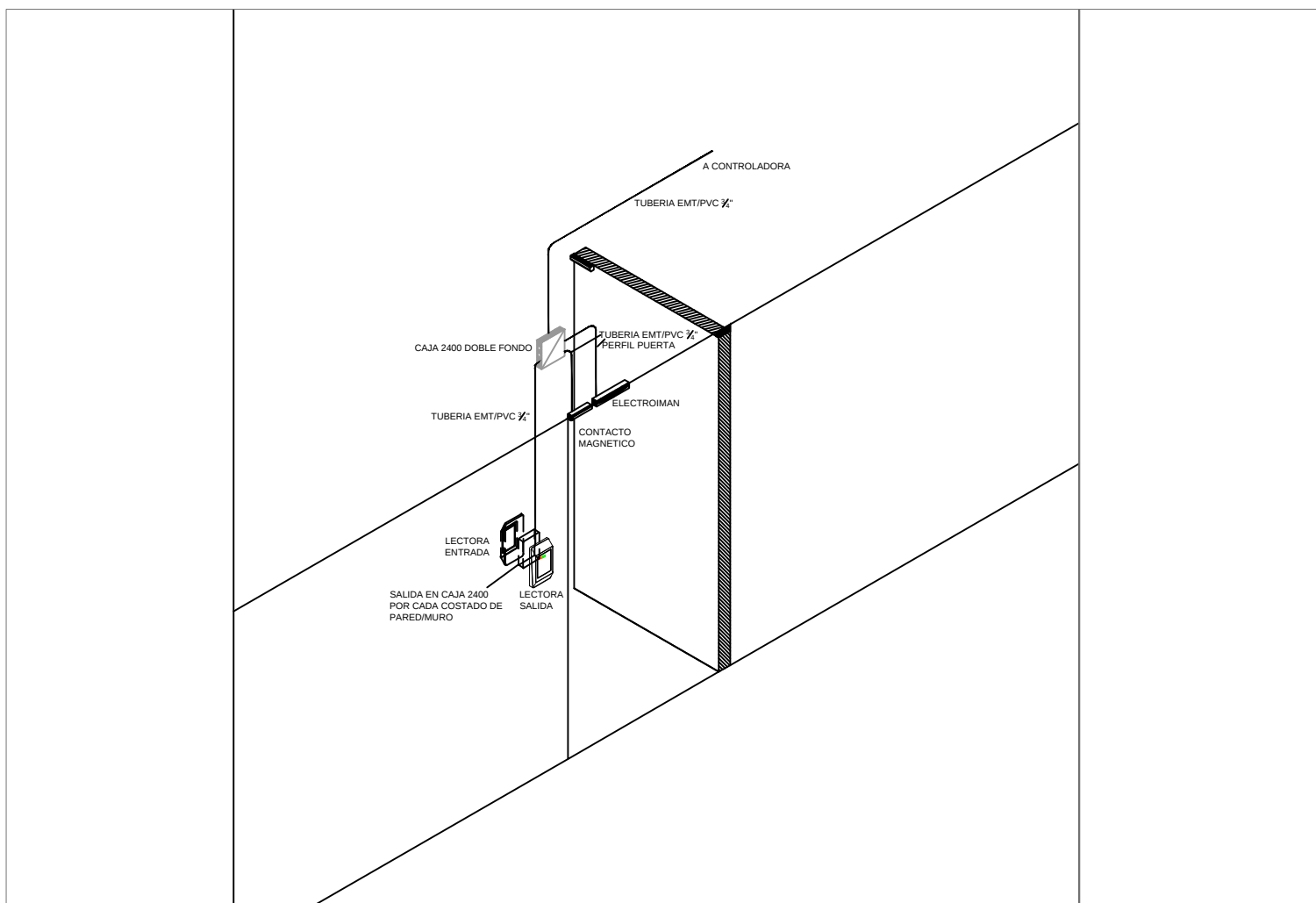
PUERTA MODELO LECTORA - LECTORA
