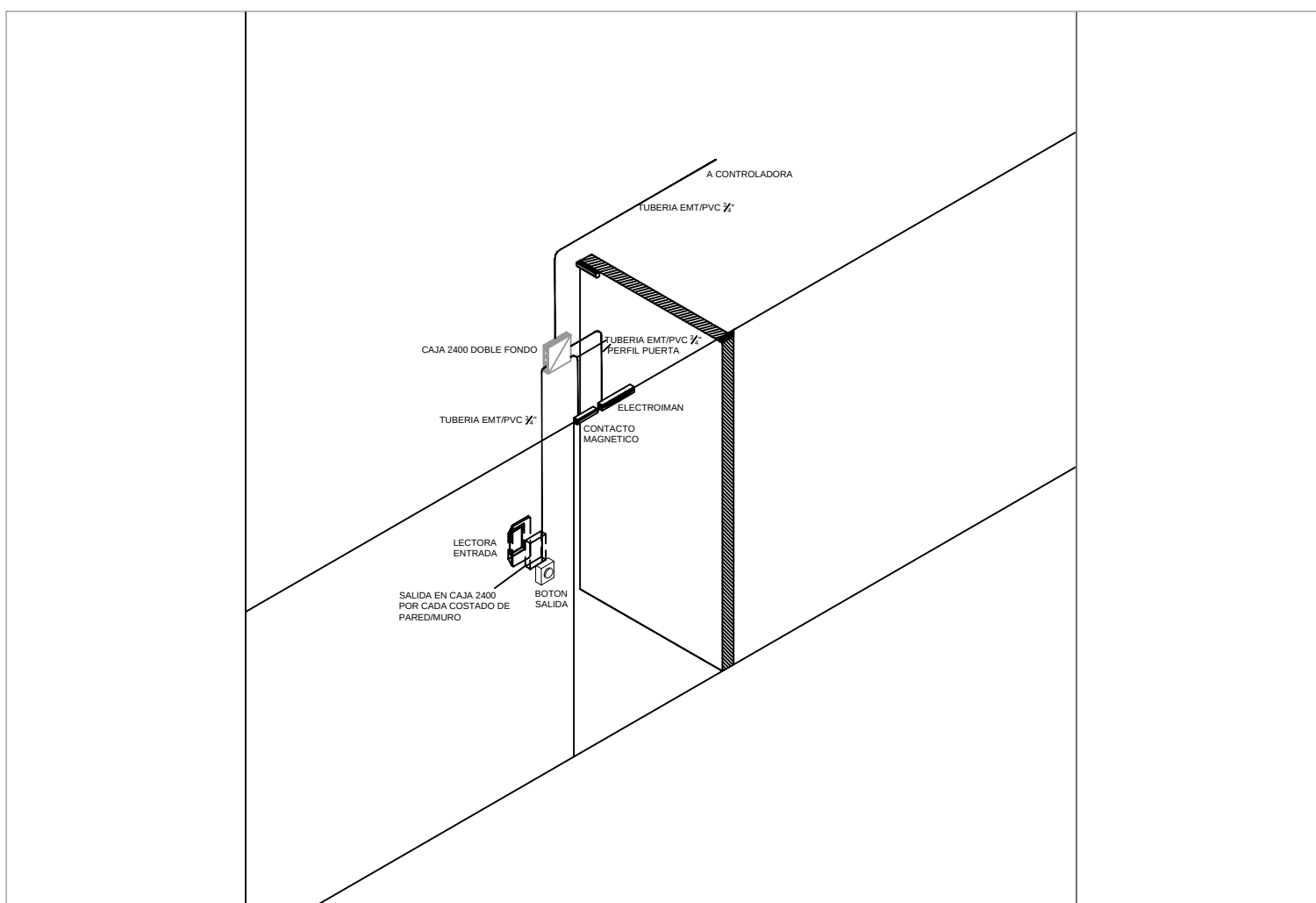
PUERTA MODELO LECTORA - BOTON
