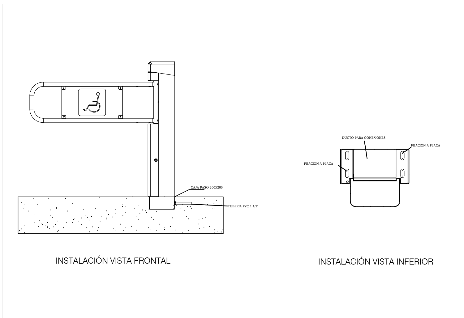
MOLINETE PERSONAS CON DISCAPACIDAD
